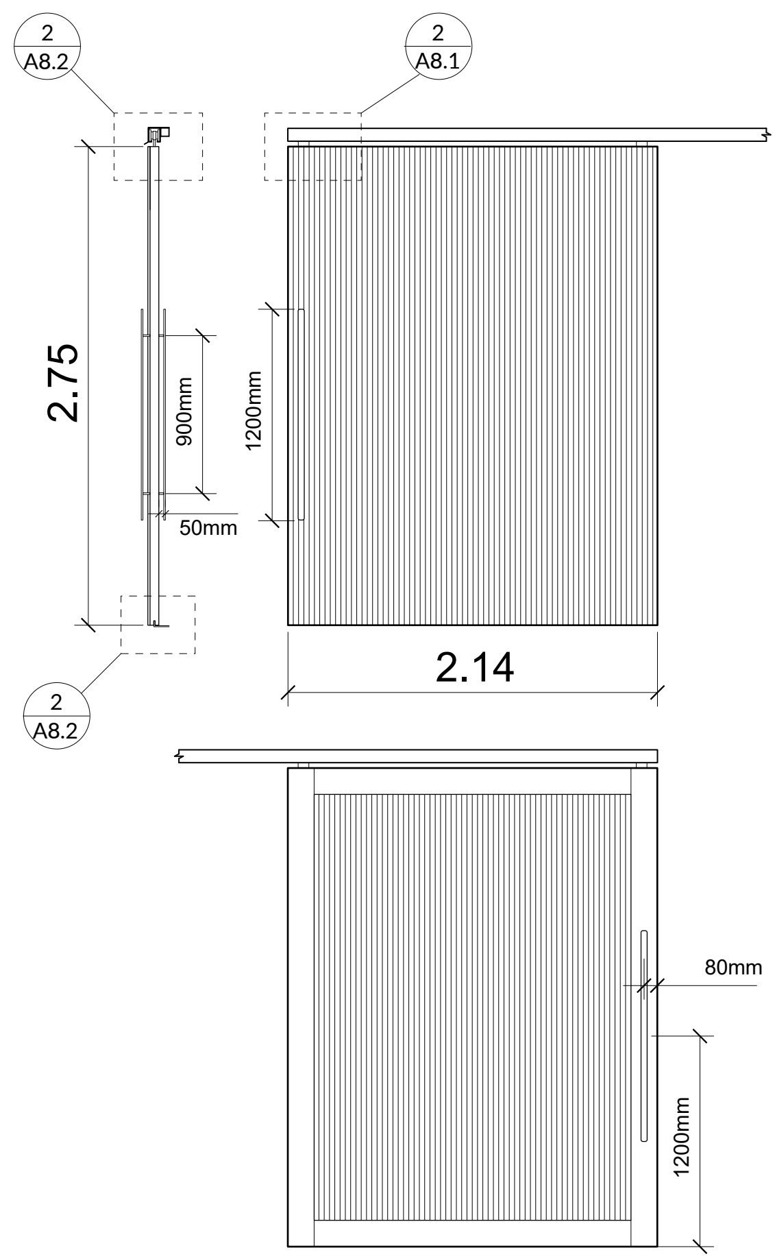
1 Elevation 1:30 Barn Door, Typ.
